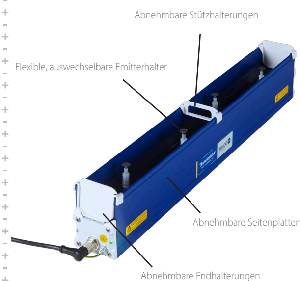
Zeichnung ThunderION IQ 2.0
